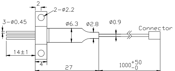
Horizontal Flange
