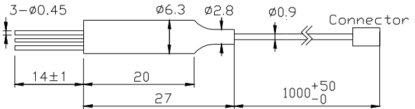
Flangeless
